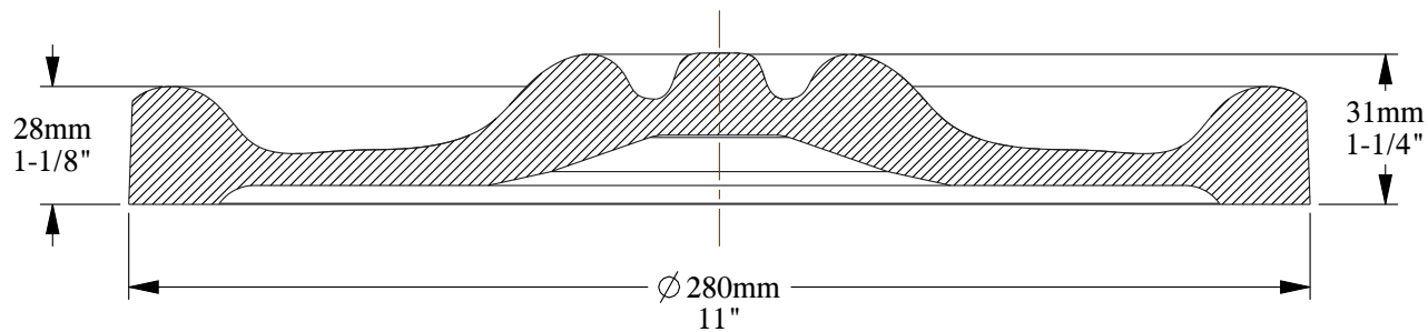
SECTION A-A SCALE 1:2
