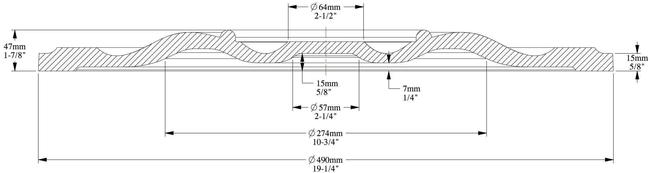
SECTION A-A SCALE 1:2
