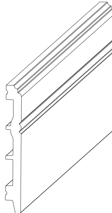
SCALE 1:2
